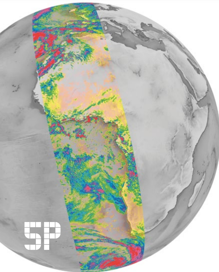
Aerosole in der Atmosphäre, aufgenommen von Sentinel-5P.
